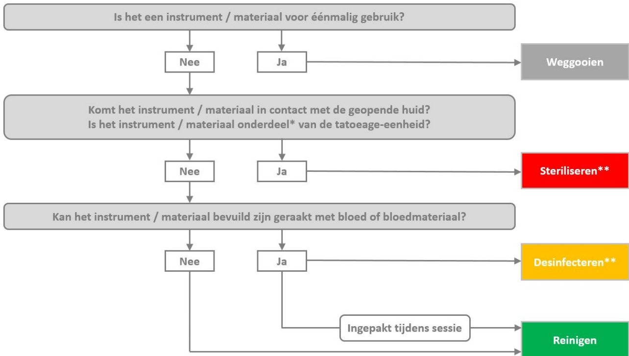
Figuur 1: geeft een stroomschema weer voor verwijderen, reinigen, desinfecteren en steriliseren.
